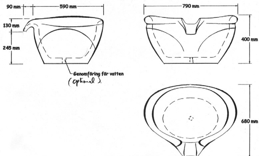
Stensund Fontän inloppskar, vit slätbetong
